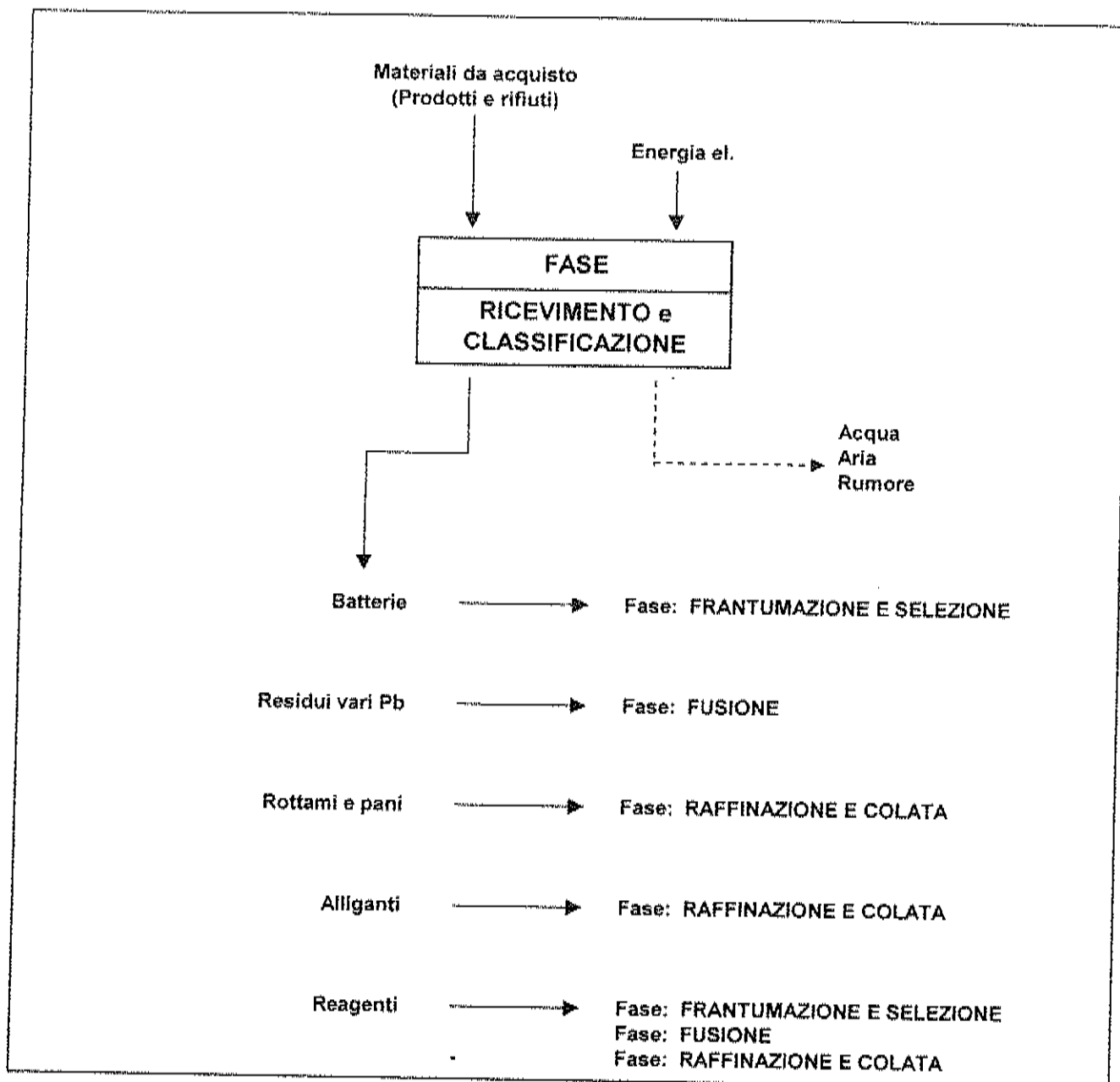
Figura B.2 Schema di flusso ricevimento e classificazione
