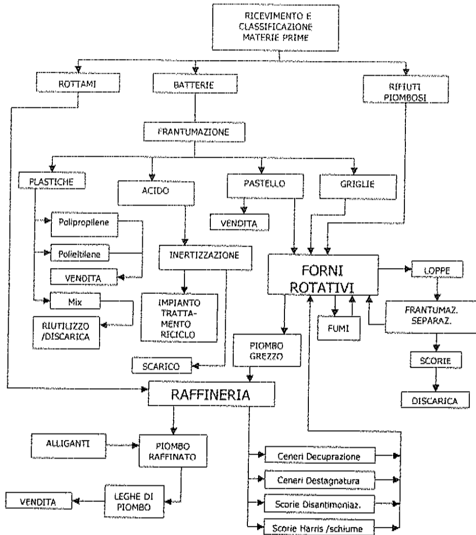
Figura B.1 Schema di flusso dell'intero ciclo
