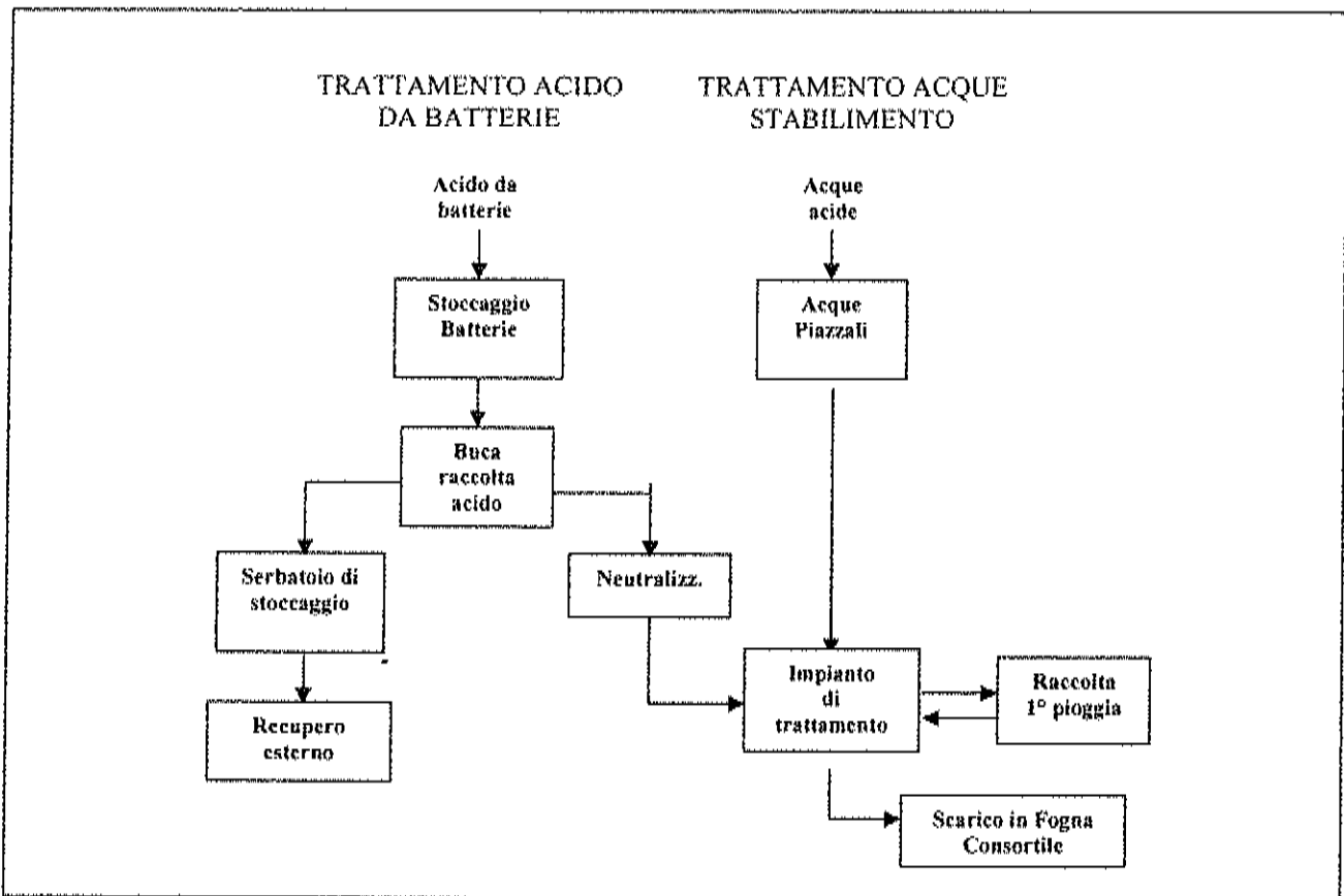
Figura C.1 Schema di flusso dell'impianto di trattamento acque
